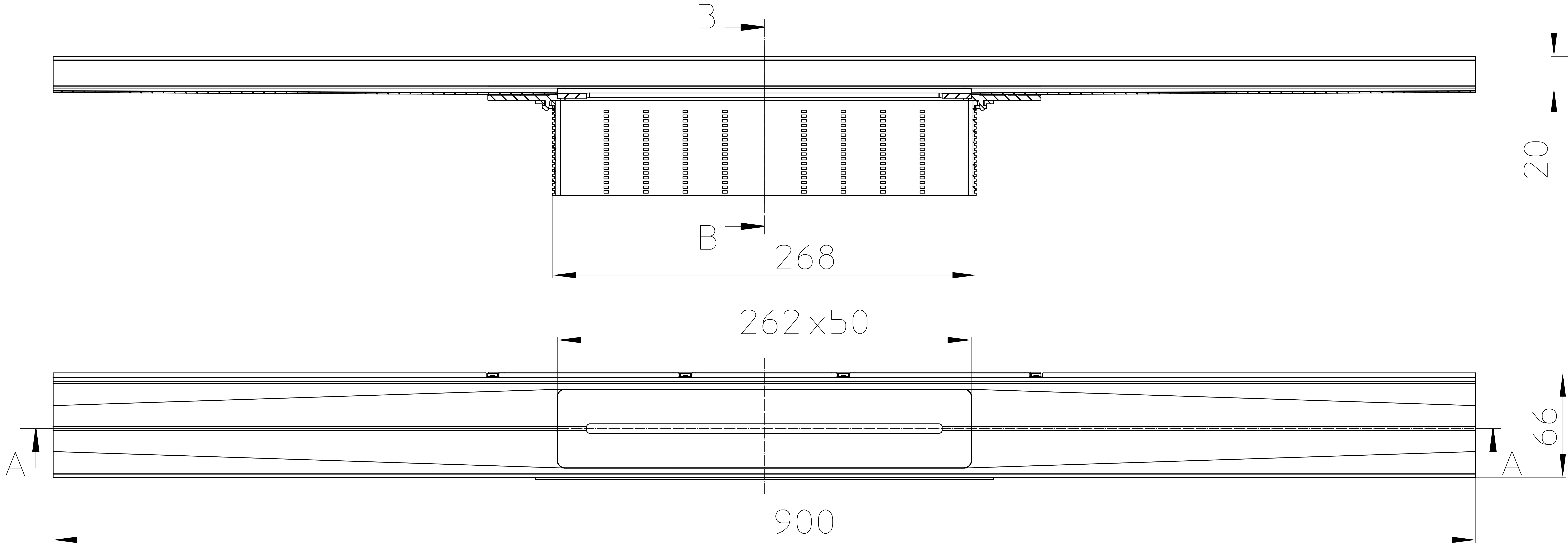
Schnitt A-A
